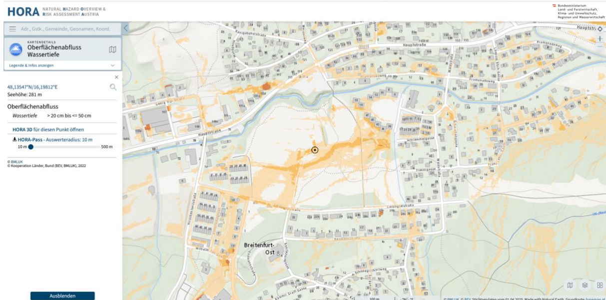
Abbildung 2. Oberflächenabfluss-Karte für das Projektgebiet „Wiesenpark Breitenfurt“, punktuell hervorgehoben sind die Wassertiefen für die orange-markierten Bereiche ( > 20 \text{ cm} < 50 \text{ cm} ); Datengrundlage: hora.gv.at .
