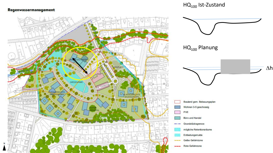
Abbildung 1. Planische Darstellung des „Wiesenparks Breitenfurt“ (Hawlik Gerginski Architekten ZT GmbH) überlagert mit der roten und gelben Zone im Ist-Zustand; ergänzende Darstellung der Auswirkungen der Verbauungen im HQ 100 -Abflusskorridor.
