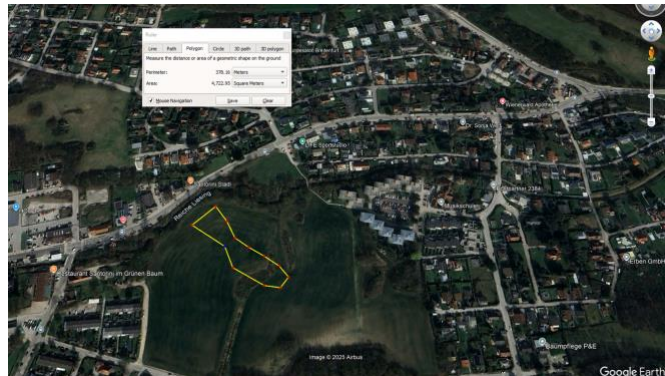
Abbildung 3. (a) geplante Flutmulde, bzw. Ableitungsstränge im Bereich des „Wiesenparks Breitenfurt“, (b) Abschätzung der Größe der geplanten Flutmulde mittels GoogleEarth.
